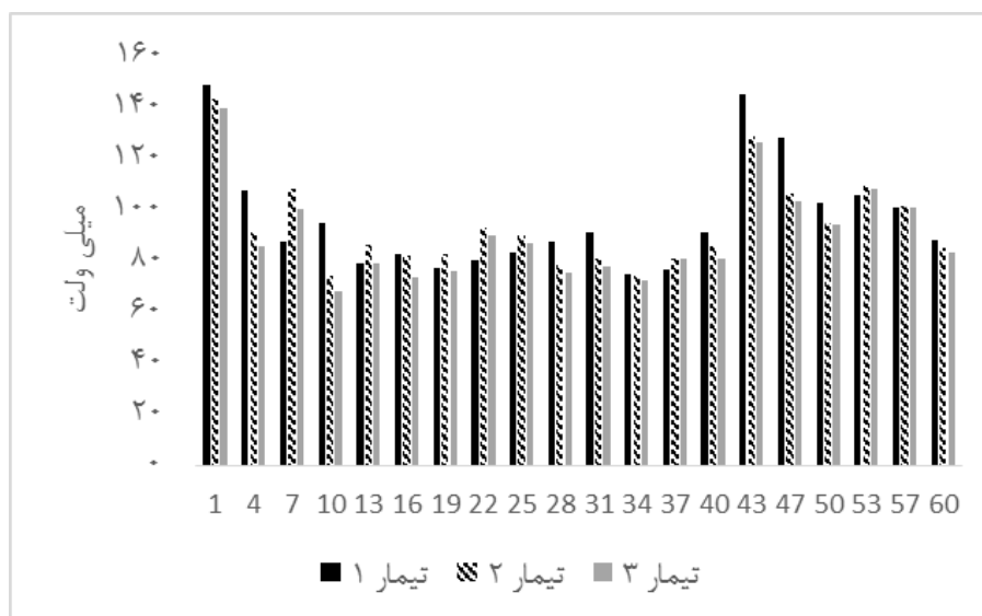
شکل ۳ - تغییرات شاخص ORP در طول دوره ی ۶۰ روزه.
