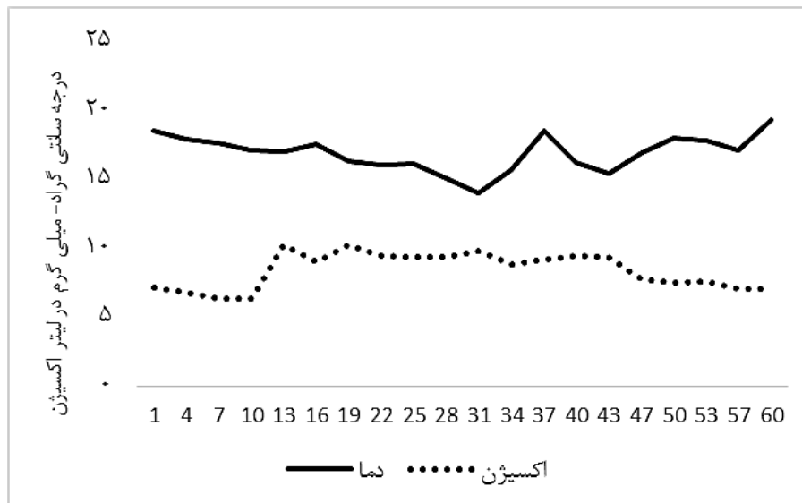
شکل ۱ - تغییرات دما و اکسیژن در طول دوره ۶۰ روزه.
