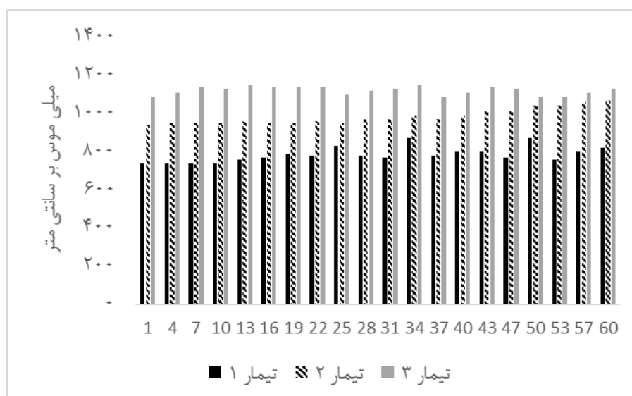
شکل ۴ - تغییرات شاخص EC در طول دوره ی ۶۰ روزه.
