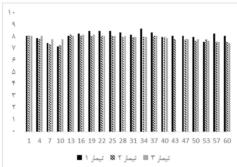
شکل ۲ - تغییرات پی اچ در طول دوره ۶۰ روزه.
