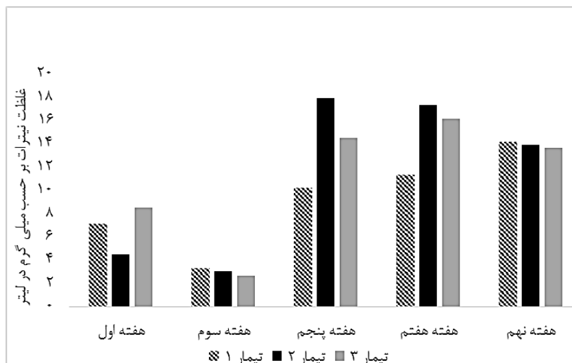
شکل ۶ - تغییرات میزان نیترات در طول دوره.
